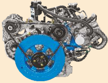
700 DI ఇంజన్ వాటర్ కూల్డ్ ఇంజన్
